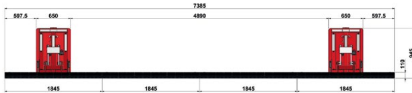
Sperrre mit vier Elementen: zwei geschlossene, zwei abgesenkte. Durchfahrtsbreite: 4,9 Meter.
