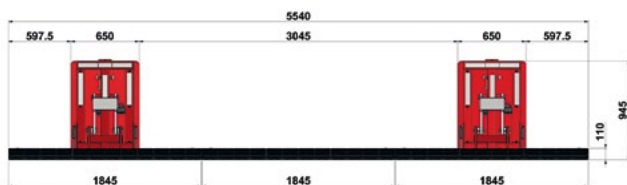
Sperrre mit drei Elementen: zwei geschlossene, ein abgesenkte. Durchfahrtsbreite: 3 Meter.
