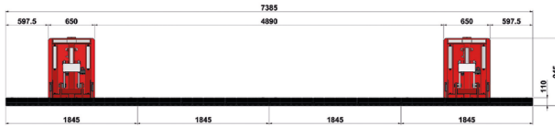
Sperre mit vier Elementen: zwei geschlossene, zwei abgesenkte. Durchfahrtsbreite: 4,9 Meter.
